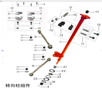
转向柱组件
