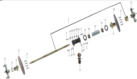
后桥总成
